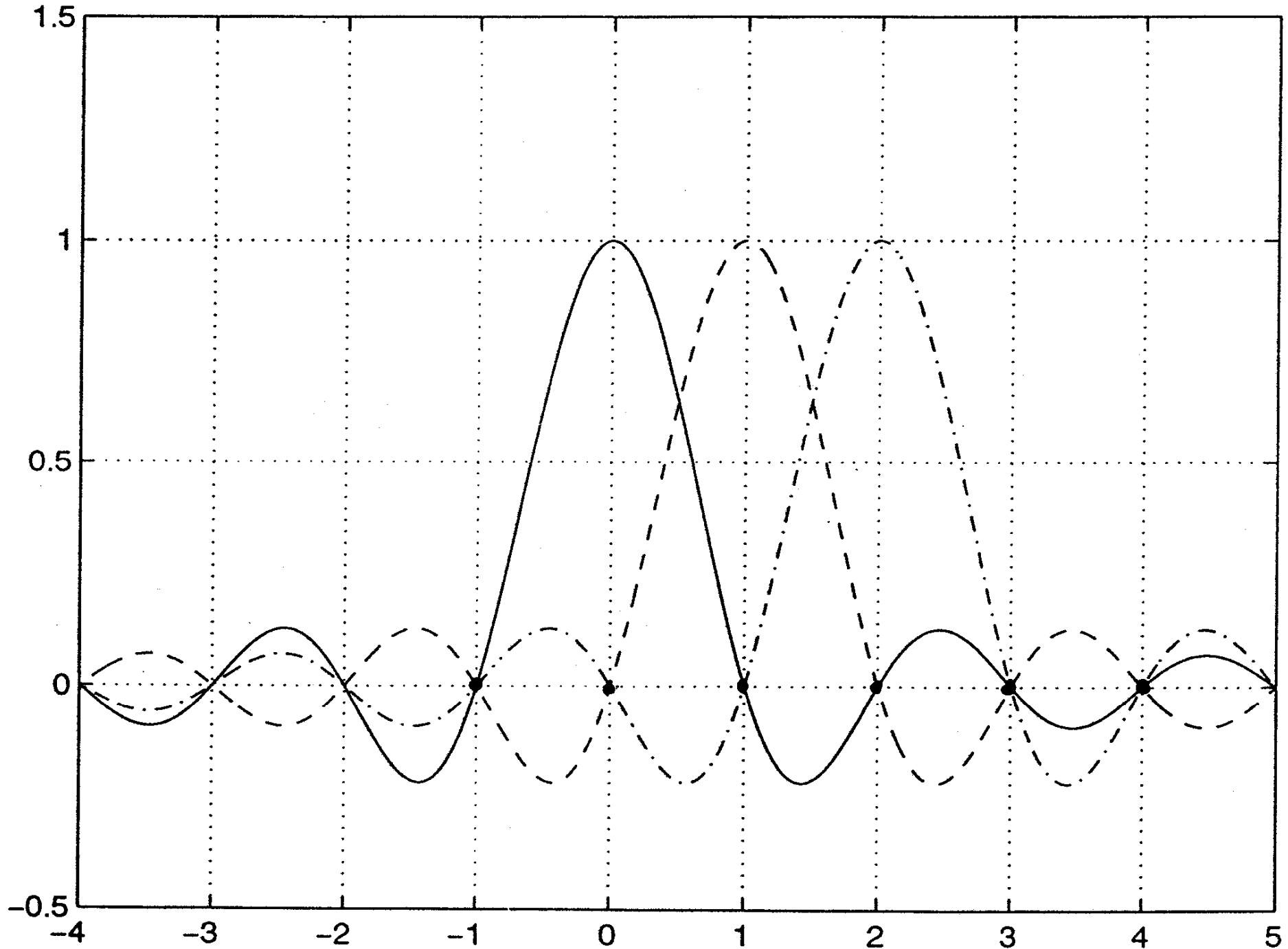
Secuencia de tres pulsos de Nyquist transmitidos
